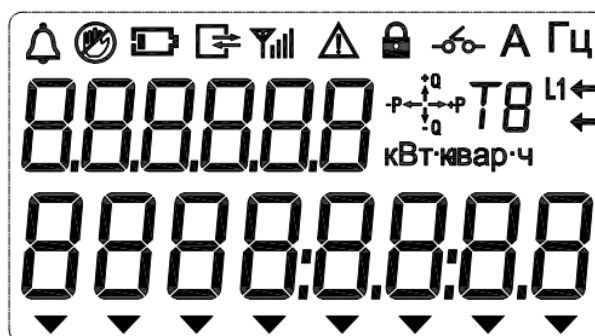
Рисунок 12 – Общий вид ЖКИ счетчика исполнения «ХК»
