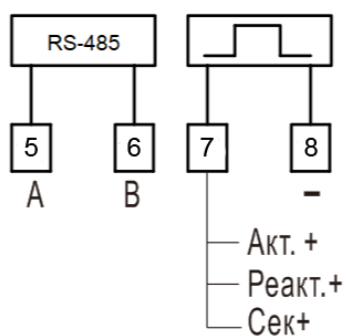
Рисунок 7 - Схема дополнительных зажимов счетчика исполнения «ХК»
