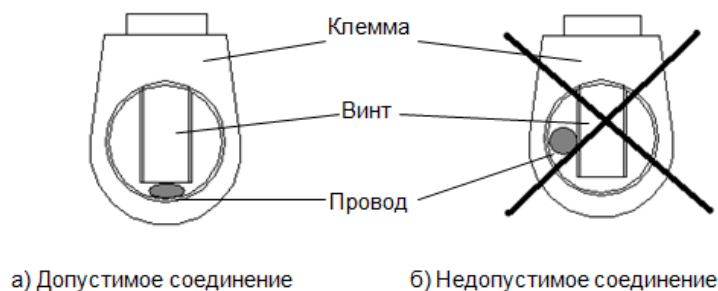
Рисунок 417 – Расположение провода в винтовой клемме при подключении счетчика
