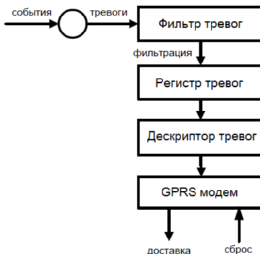
Рисунок 31 – Формирование инициативной передачи (Push)
