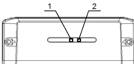
Рисунок 8 - Положения светодиодов состояния коммуникационного модуля счетчика исполнения «Х»
