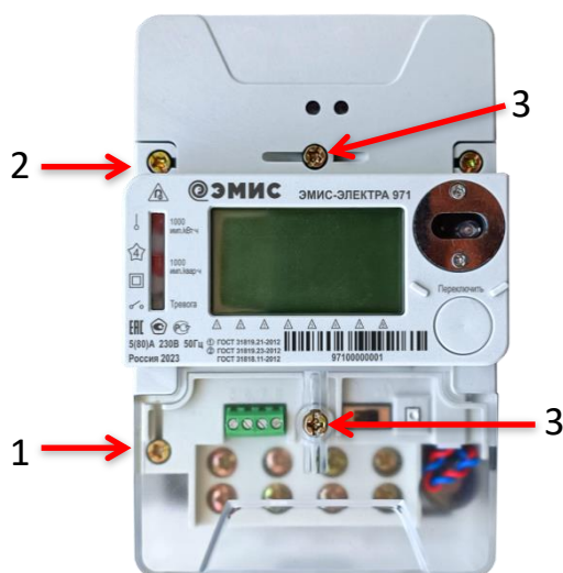
Рисунок 45. Места установки контрольных пломб счетчика исполнения «ХК»
