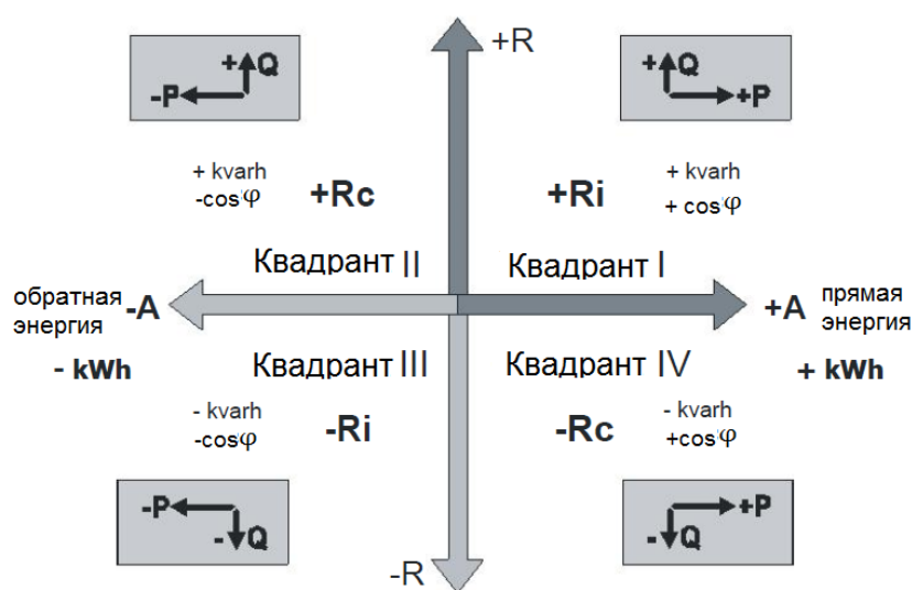
Рисунок 26 – Энергия и мощность в 4-х квадрантах
