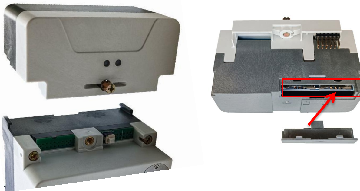
Рисунок 137 – Внешний вид и установка SIM-карты в слот БВПД счетчика исполнения «ХК»
