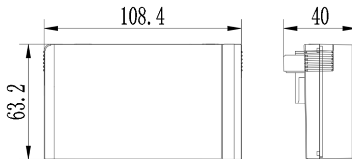
Рисунок Б.2 - Габаритные размеры коммуникационного модуля PLC / RF / PLC+RF счетчика исполнения «Х»
