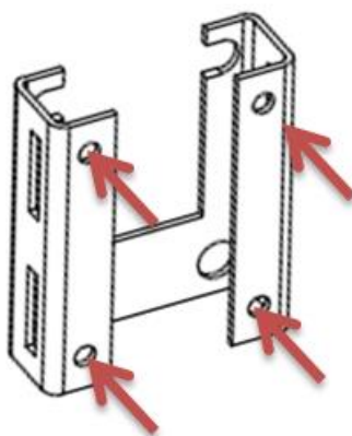
Рисунок 37 – Места крепления кронштейна для счетчика исполнения «С»
