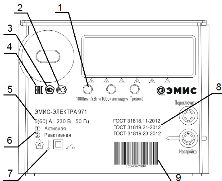
Рисунок 439 - Вид щитка счетчика исполнения «Х»
