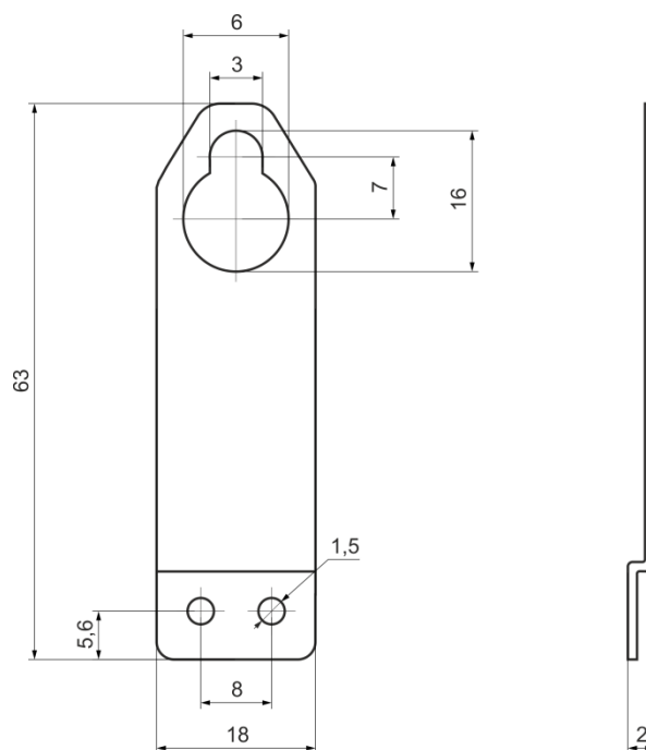
Рисунок В.2 - Габаритные размеры крепежной проушины для счетчика исполнения «JK»
