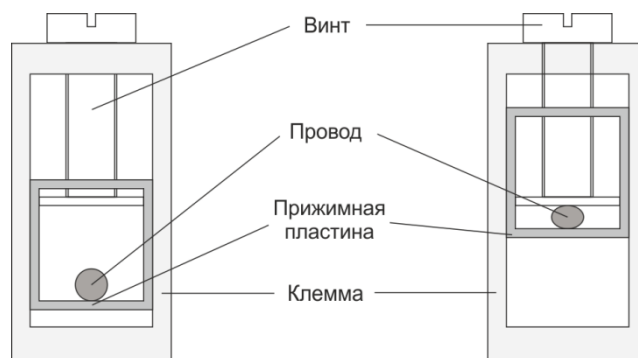
Рисунок 428 – Расположение провода в клемме с прижимной пластиной при подключении счетчика
