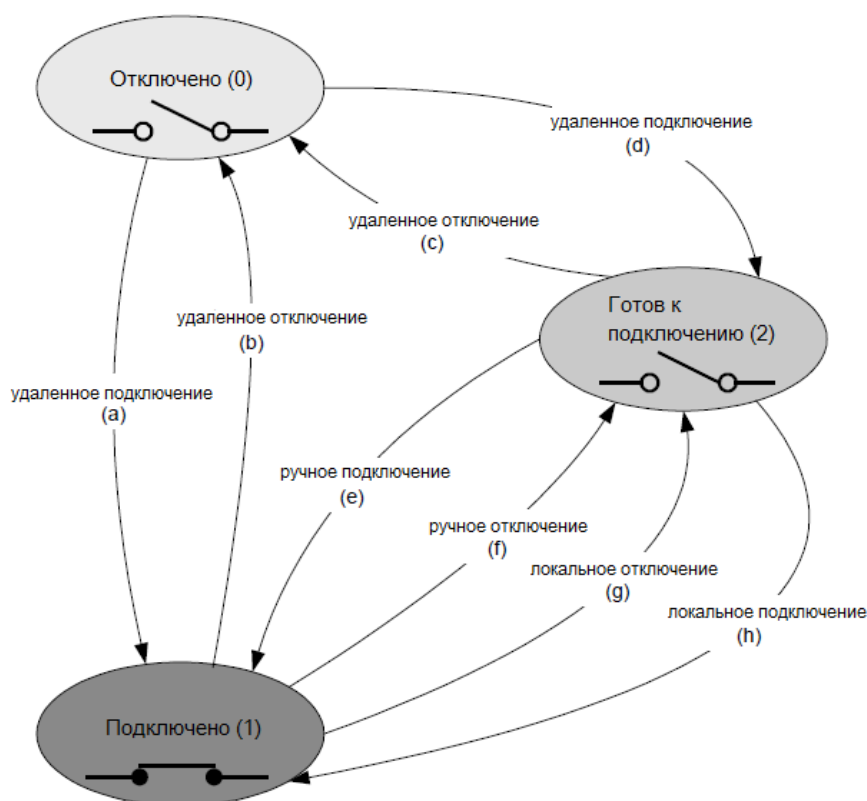
Рисунок 27 - Основные переходы состояния реле
