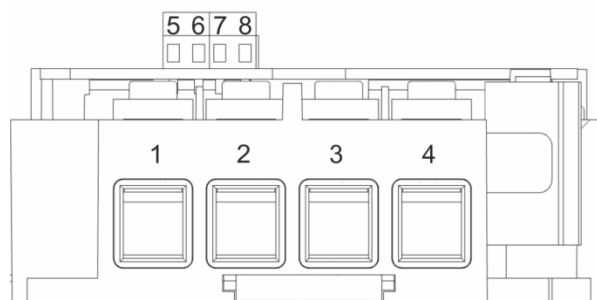
Рисунок 6 – Вид отсека зажимов счетчика исполнения «ХК»
