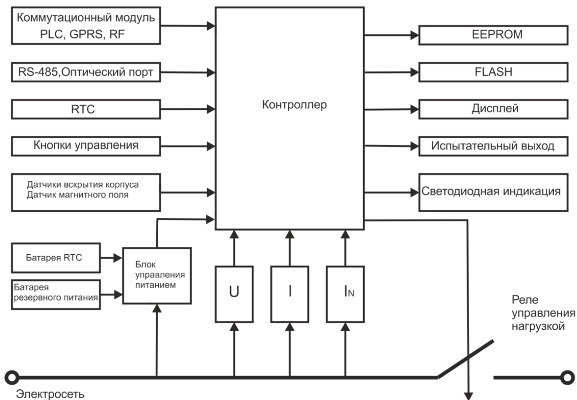
Рисунок 9 – Структурная схема счетчика исполнения «Х» и «ХК»
