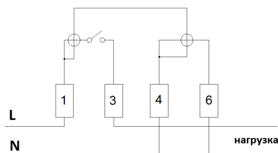
Рисунок 406 – Схема подключения счетчика ЭМИС-ЭЛЕКТРА 971
