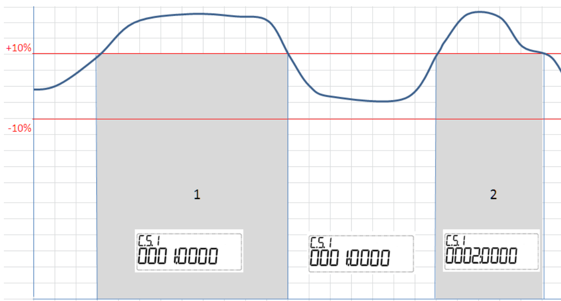
Рисунок 3721 - Пример фиксирования события нарушения качества напряжения
