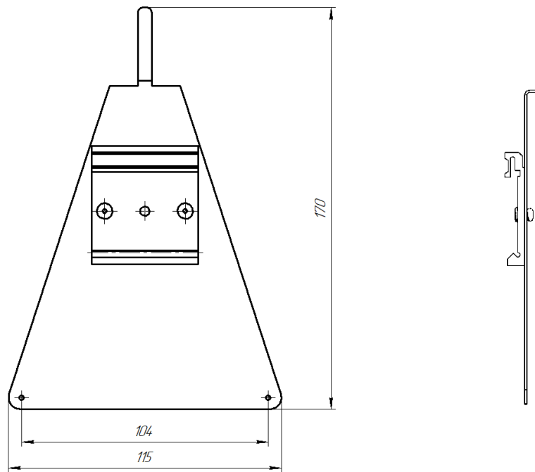
Рисунок В.3 - Габаритные размеры крепежного кронштейна для счетчика исполнения «Х»
