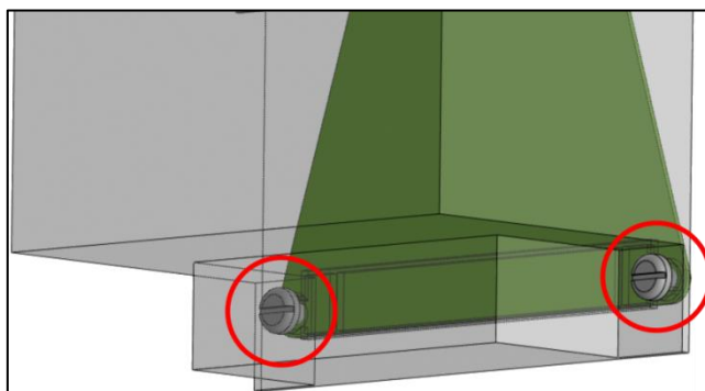
Рисунок 38 – Крепление счетчика исполнения «Х» на монтажной рейке
