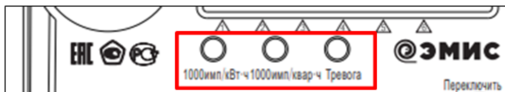
Рисунок 15 – Общий вид индикаторов состояния счетчика исполнения «Х»
