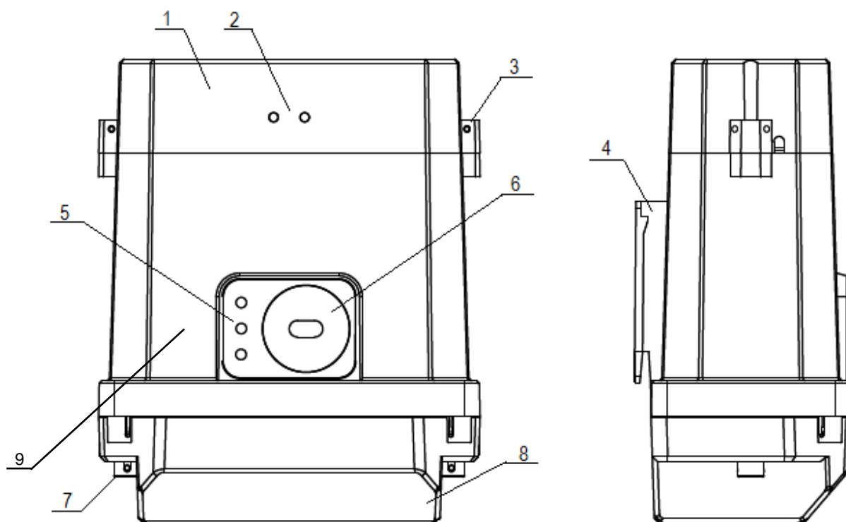
Рисунок 2 - Общий вид счетчика исполнения «С»
