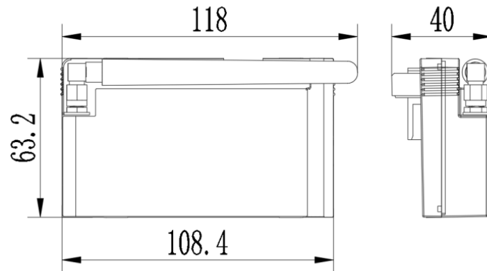
Рисунок Б.1 - Габаритные размеры БВПД GPRS / NB-IoT / LoRaWAN счетчика исполнения «Х»
