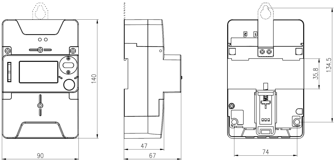
Рисунок А.3 - Габаритные размеры и установочные размеры счетчика ЭЭ-971 исполнения «ХК»
