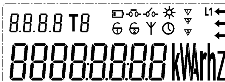
Рисунок 3 – Общий вид дисплея дополнительного устройства индикации
