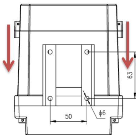
Рисунок 395 – Крепления счетчика исполнения «С» на кронштейне
