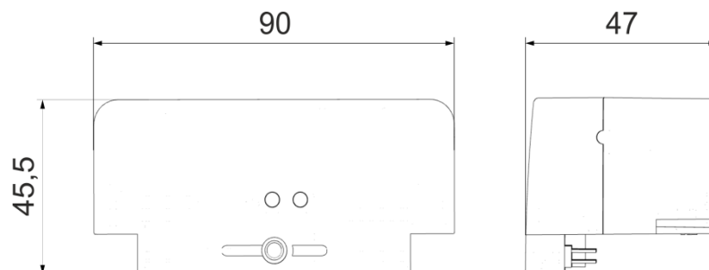
Рисунок Б.3 - Габаритные размеры БВПД счетчика исполнения «ХК»
