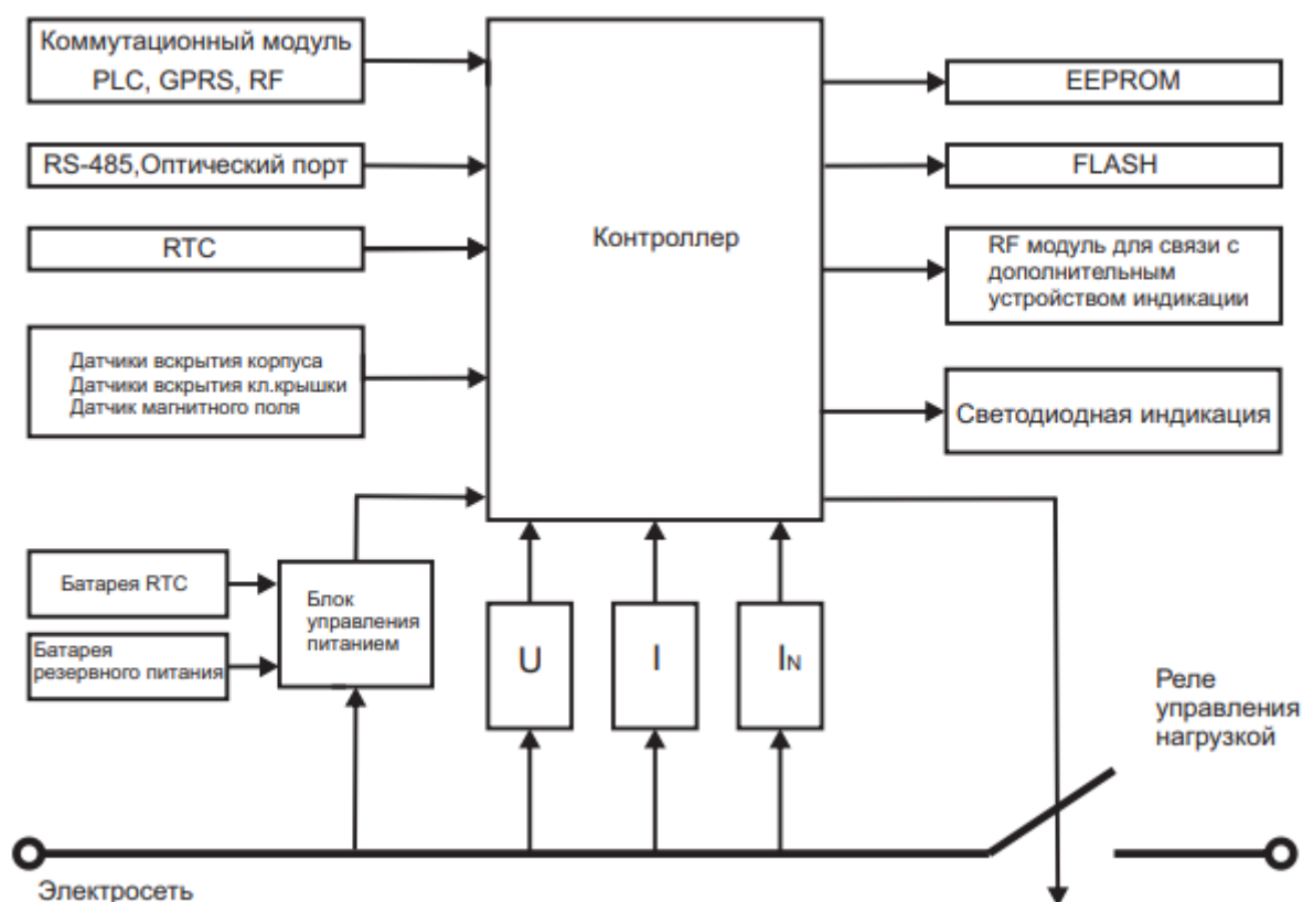
Рисунок 10 – Структурная схема счетчика исполнения «С»
