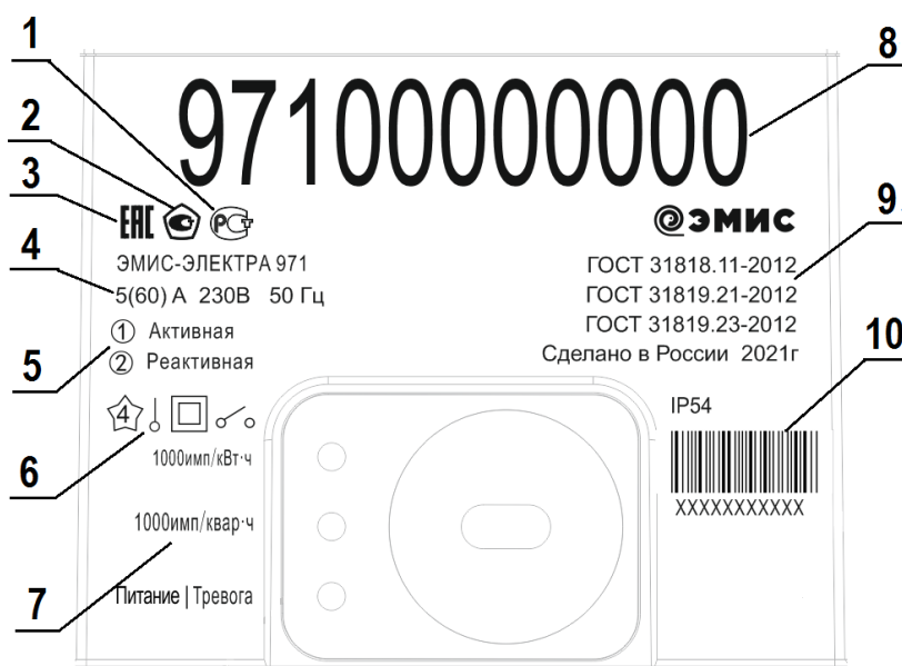
Рисунок 44 - Вид щитка счетчика исполнения «С»
