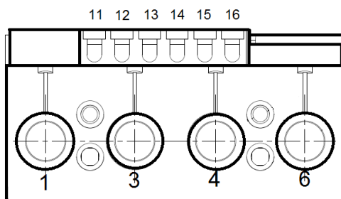
Рисунок 4 – Вид отсека зажимов счетчика исполнения «Х»
