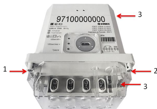
Рисунок 464. Места установки контрольных пломб счетчика исполнения «С»
