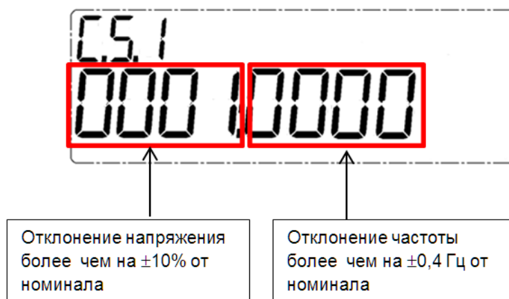
Рисунок 36 - Пример отображения события нарушения качества напряжения
