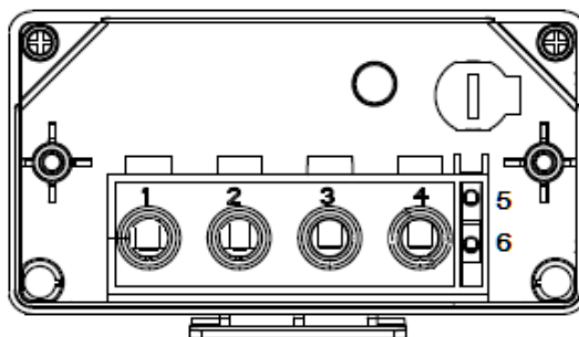
Рисунок 8 – Вид отсека зажимов счетчика исполнения «С»
