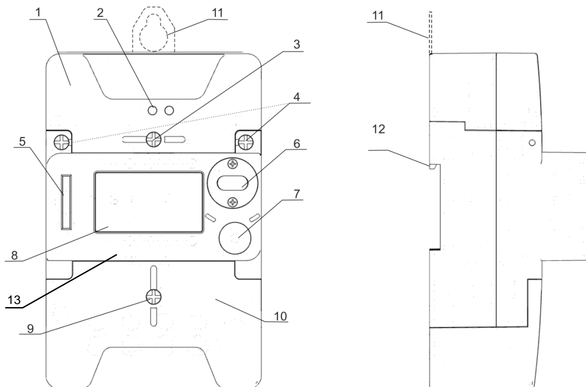
Рисунок 3 - Общий вид счетчика исполнения «ХК»
